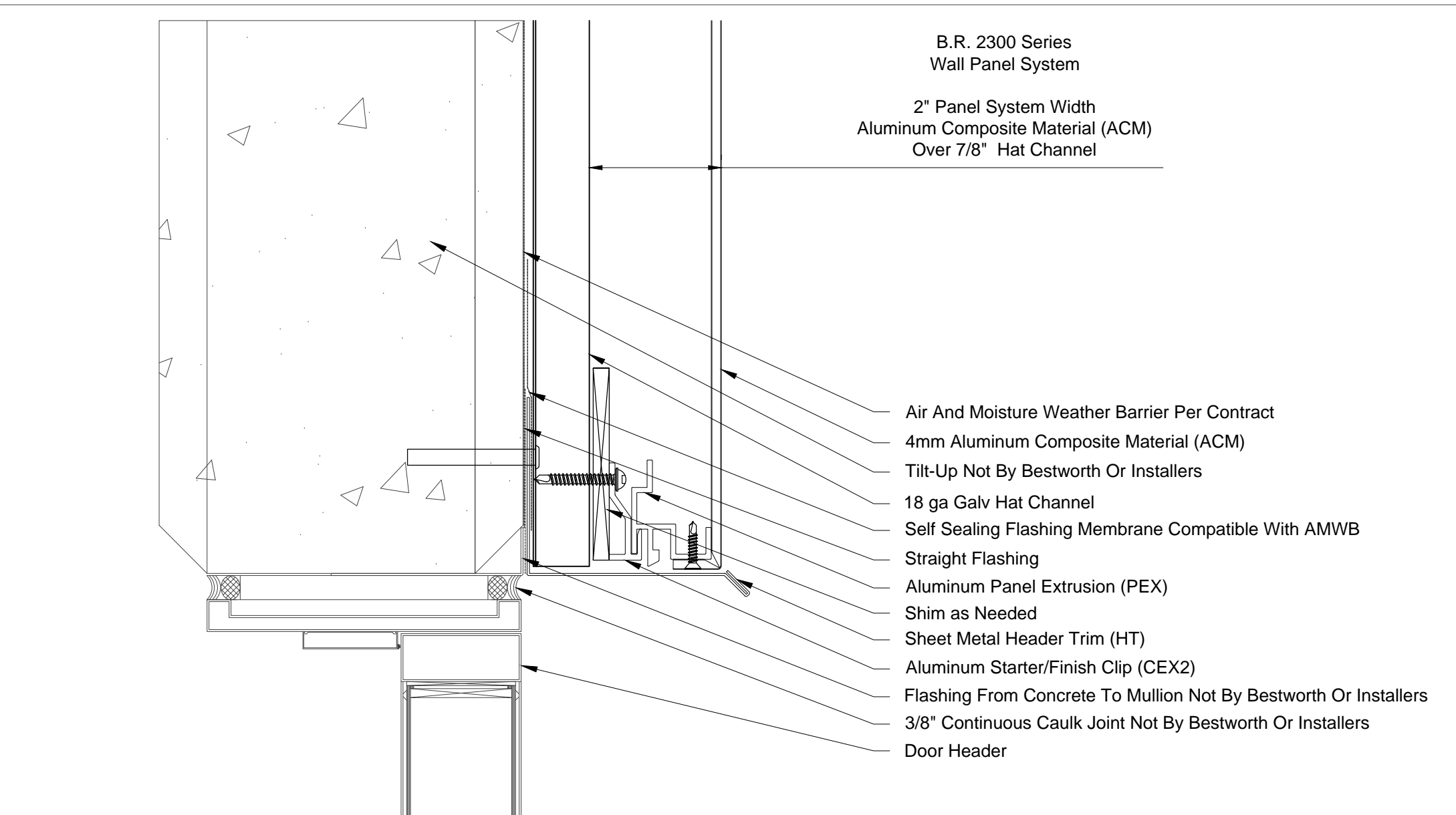
10 2300 ACM @ Door Header - Tilt Up 6" = 1'-0"
